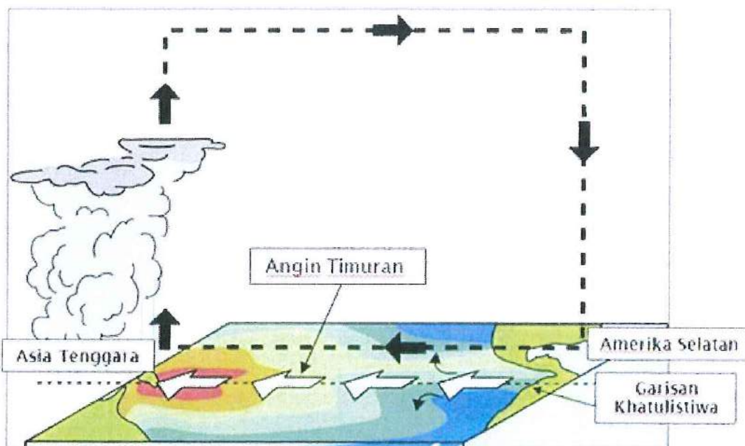
Rajah menunjukkan interaksi antara lautan dan atmosfera di Lautan Pasifik sekitar Khatulistiwa semasa Fenomena La Nina
